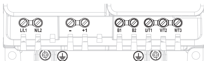
Model: HV35UB018□
