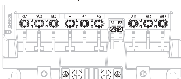
Models: HV35U2070□, 2082
