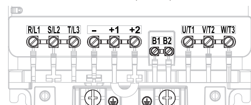
Models: HV35U4044□, 4060
