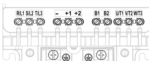
Models: HV35U2070□, 2082
