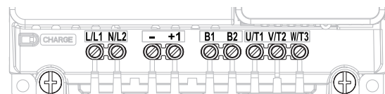
Model: HV35UB018□
