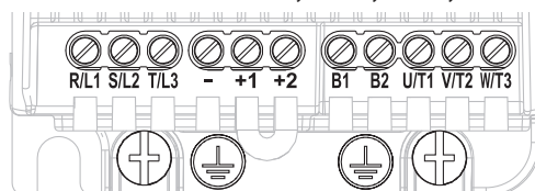
Models: HV35U2012□, 4001, 4002, 4004, 4005, 4007, 4009
