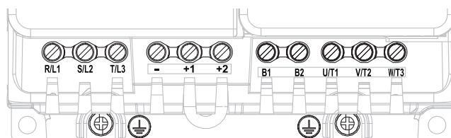
Models: HV35U2030□, 2042, 4018, 4023
