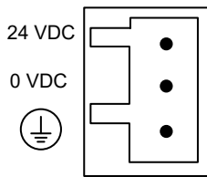
IO2310 Module
