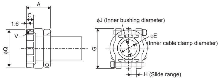
(d) MS3057A-□□A Cable Clamp with Rubber Bushing Dimensional Drawings
