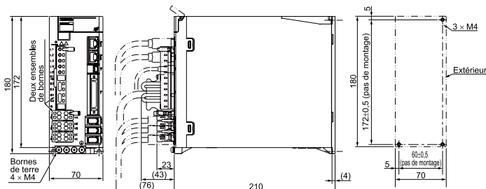
Schéma de l'orifice de montage
